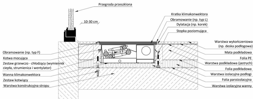
Przykład montażu klimakonwektora kanałowego CVK4
