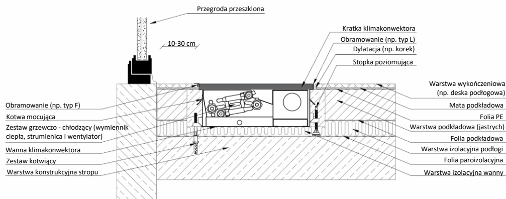
Przykład montażu czterururowego klimakonwektora kanałowego CVK4
