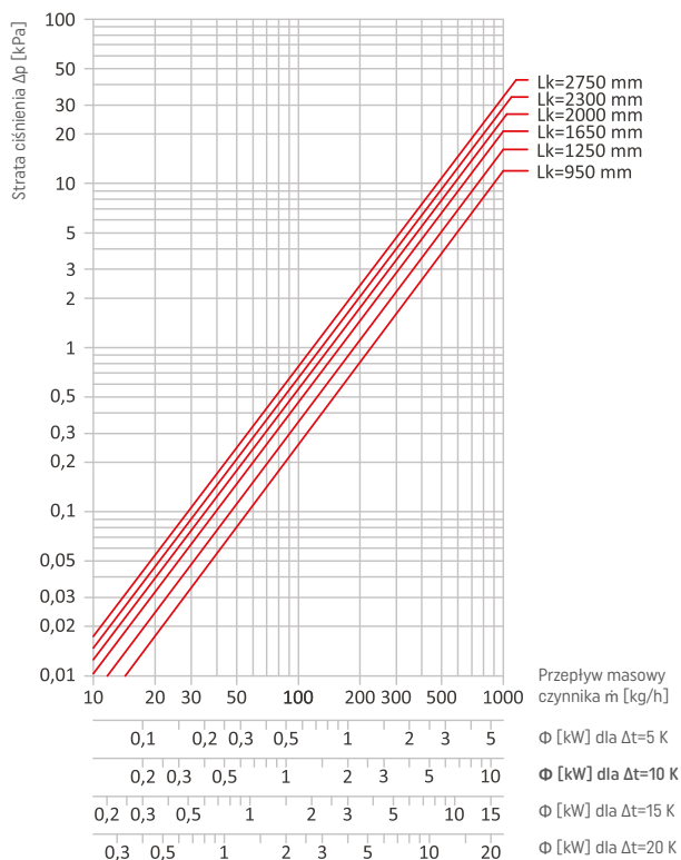
VKN5-7,5/35/Lk, VKN5-9/35/Lk
