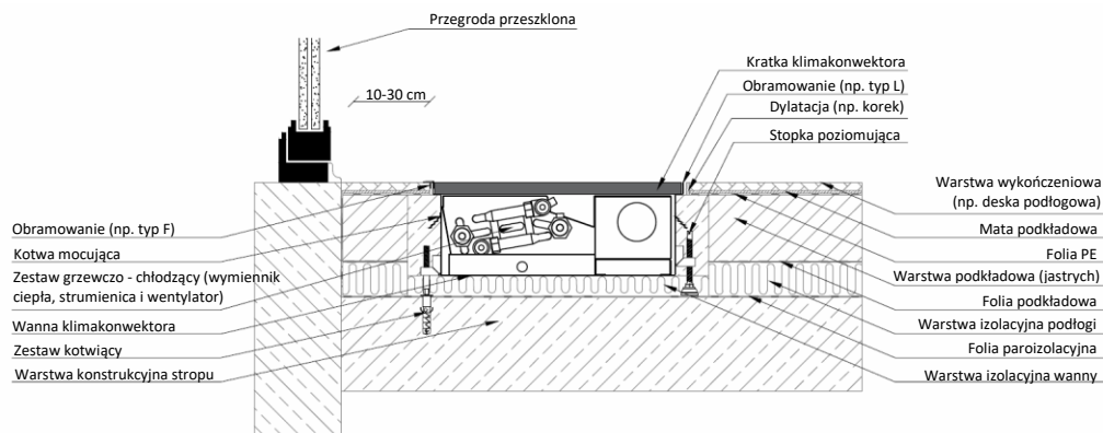
Przykład montażu czterorurowego klimakonwektora kanałowego CVK4
