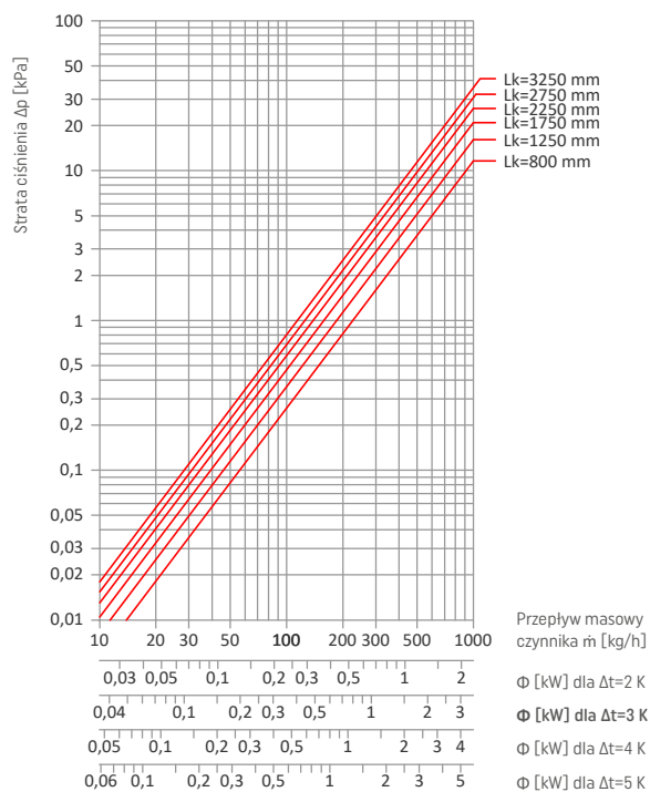
CVK4-14/29/Lk TRYB CHŁODZENIA
